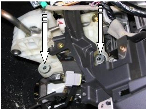
Подложить 2 шайбы
