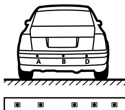
Система с 3-мя датчиками
