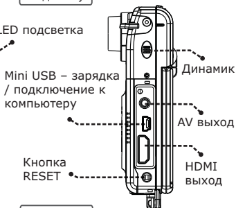
Вид сбоку
